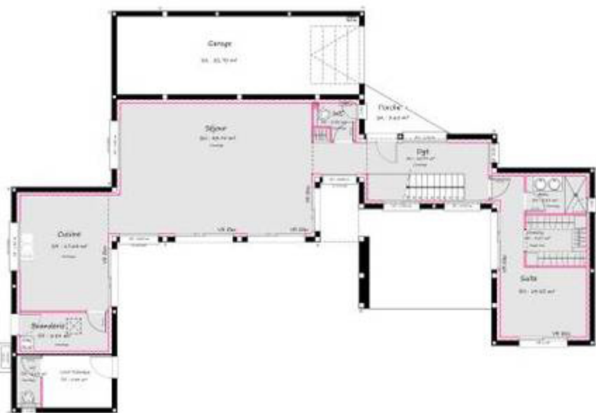
Rez-de-chaussée
