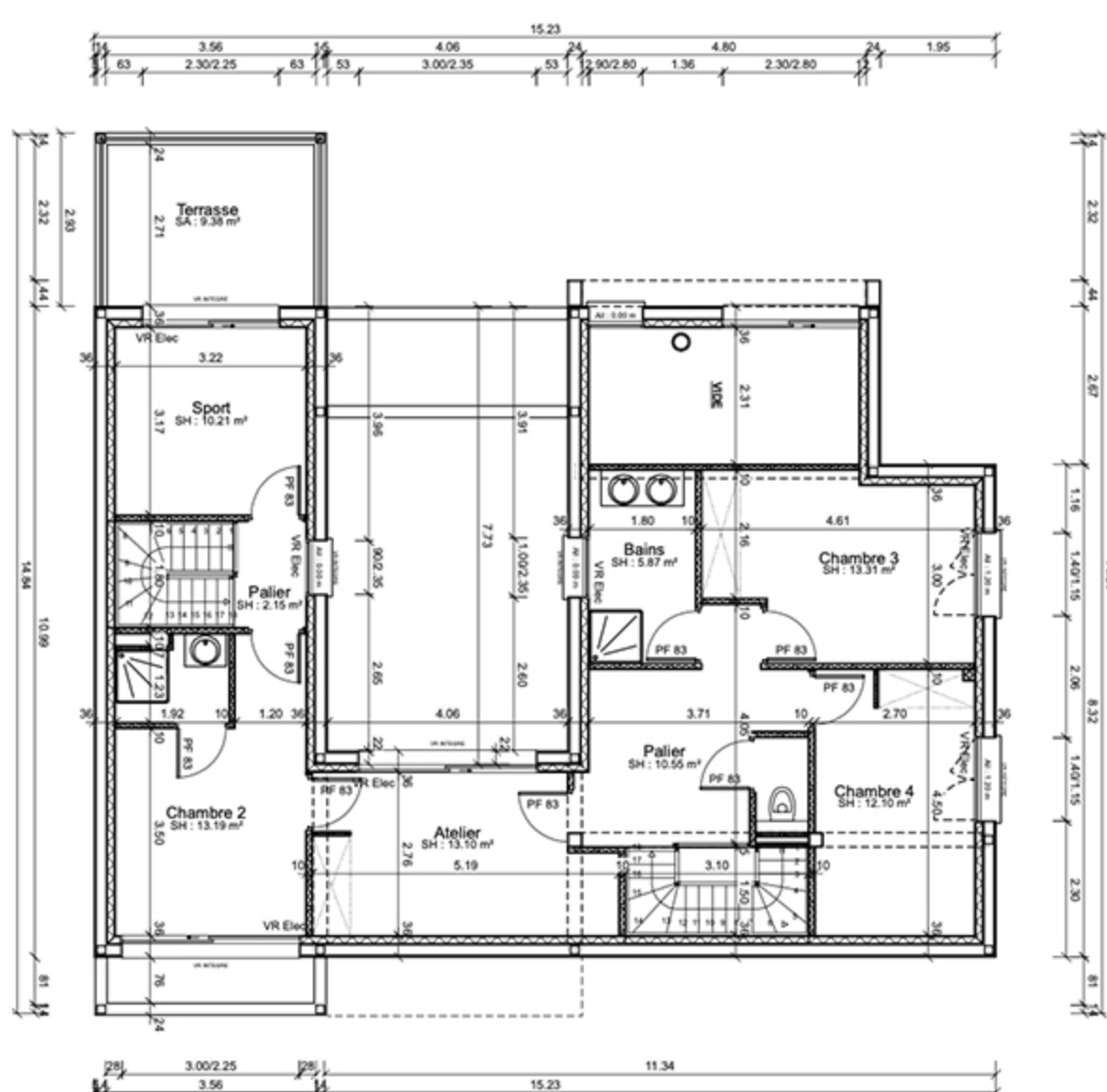
Plan de R+1
